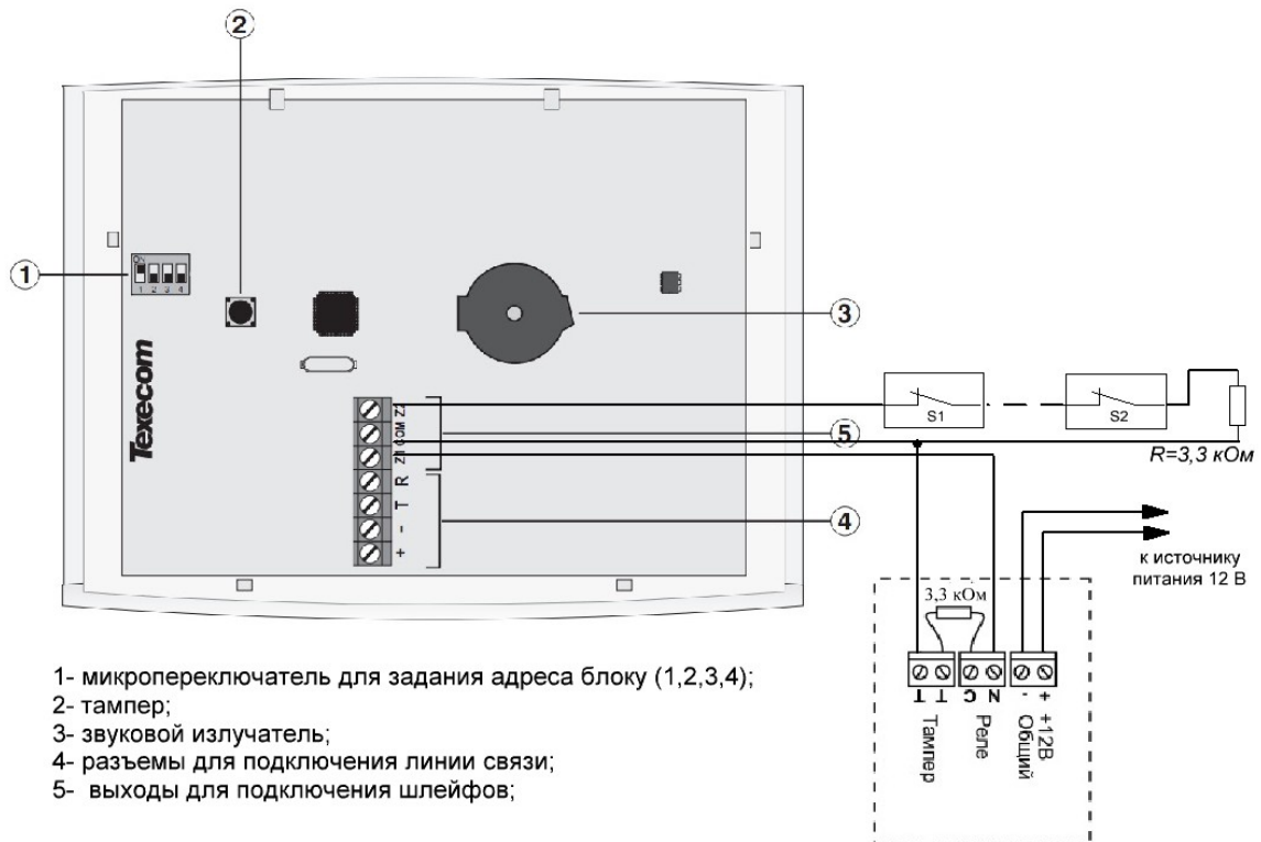
Рисунок П8 – Схема подключения шлейфов клавиатуры Texescom RKP16 PLUS
