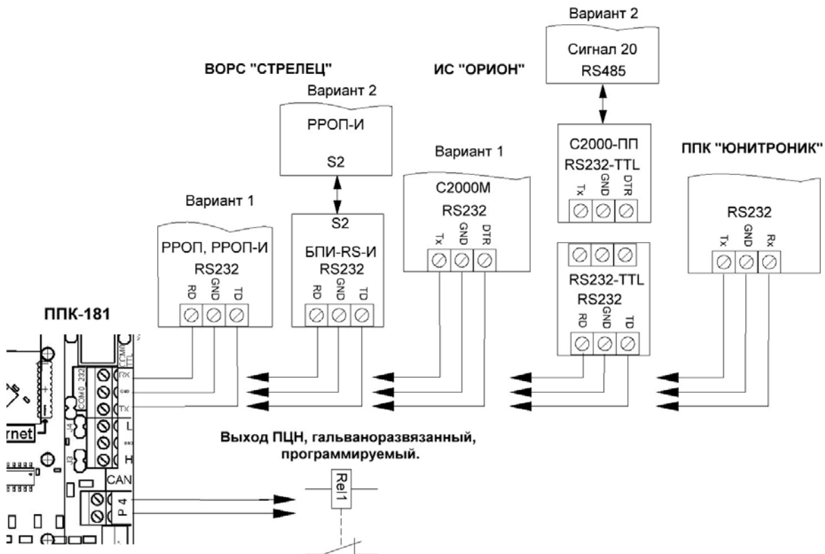
Рисунок Пб-а – Схема подключения внешних систем через интерфейс RS-232. При подключении ИС «Орион» согласно варианту 1 используется протокол обмена «ОПС «Болид»», при подключении согласно варианту 2 используется протокол «LONTA 202».
