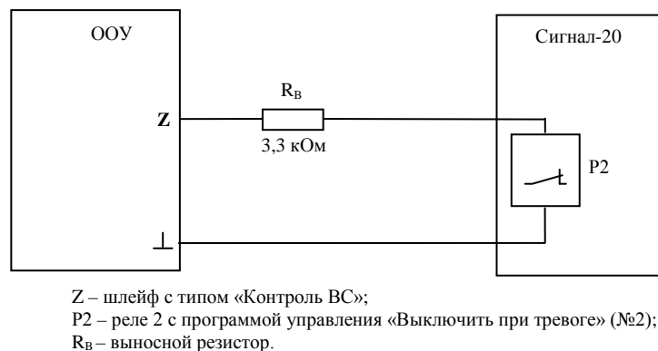
Рисунок П10 - Схема подключения прибора «Сигнал-20» через релейный выход для формирования извещений «Восстановление охранной сигнализации ВС» и «Тревога ВС».
