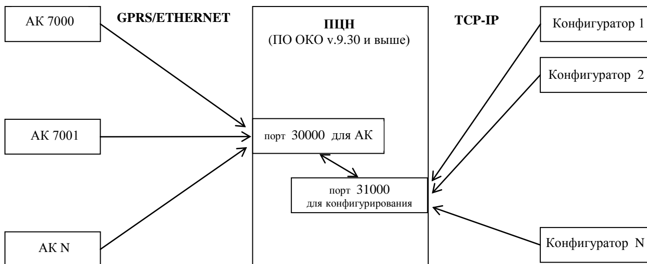
Рисунок 6.3 – Схема связи
