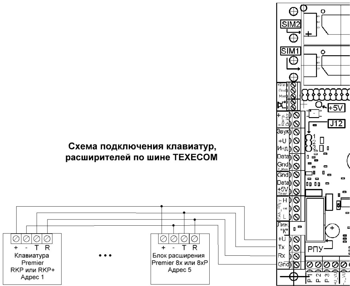
Рисунок ПЗ - Схема подключения блоков расширения TEXESOM.
