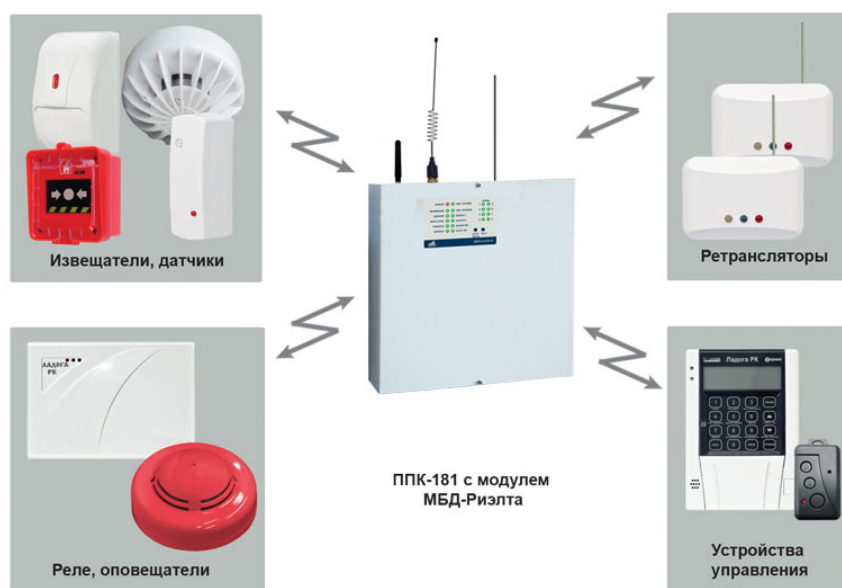
Рисунок 2.3 – Структурная схема взаимодействия ОКО-PREMIER с устройствами беспроводной системы Ладога РК
