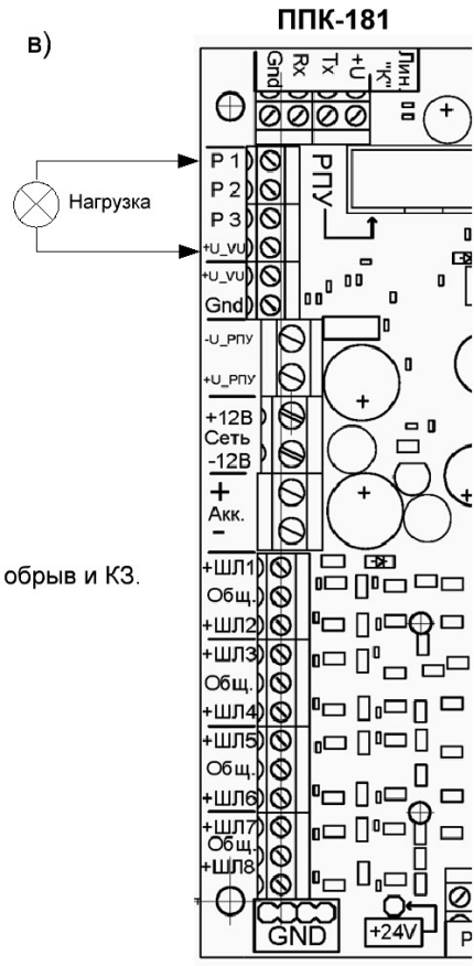
Рисунок П2 - Схема подключения к релейным выходам P1...P3.
