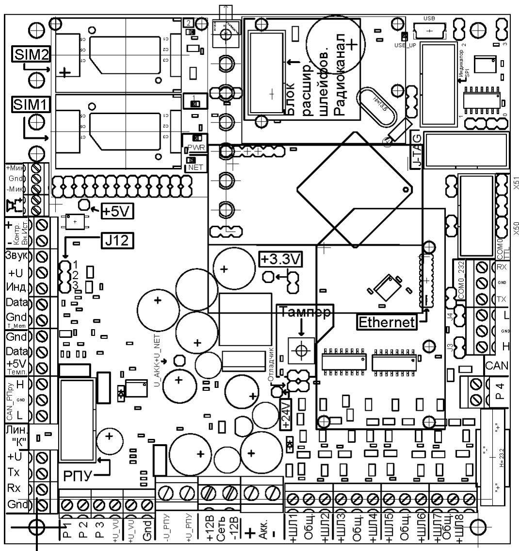
Рисунок П12 – Изображение платы ОС-181.
