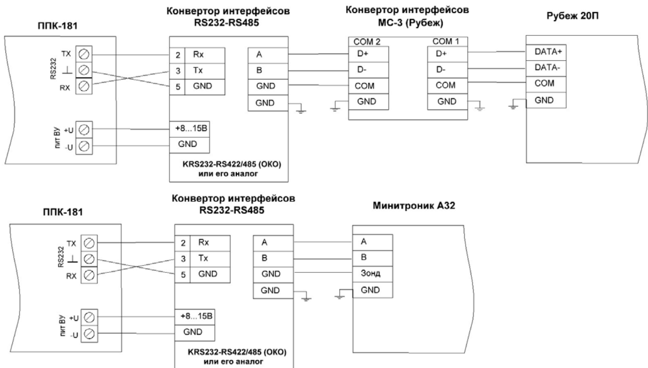
Рисунок Пб-б – Схема подключения внешних систем Рубеж 20П (протокол LONTA 202) и Минитроник А32 через интерфейс RS-485.
