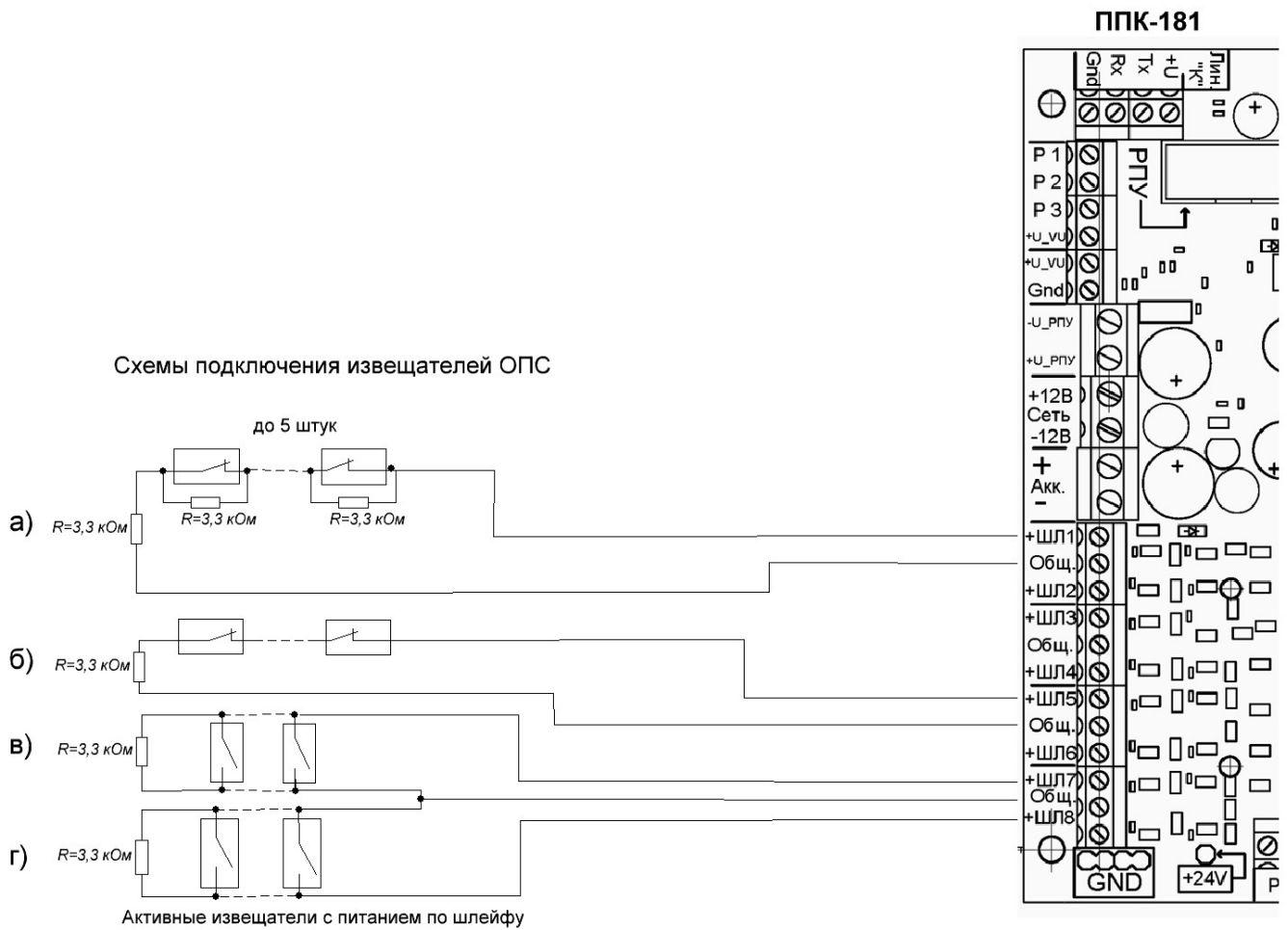
Рисунок П5 – Схема подключения датчиков к базовому блоку ОС-181. а) Шлейф с контролем 4-х состояний. б) Шлейф с контролем 3-х состояний с извещателями с нормально замкнутыми контактами. в) Шлейф с контролем 3-х состояний с извещателями с нормально разомкнутыми контактами. г) Активный пожарный извещатель.
