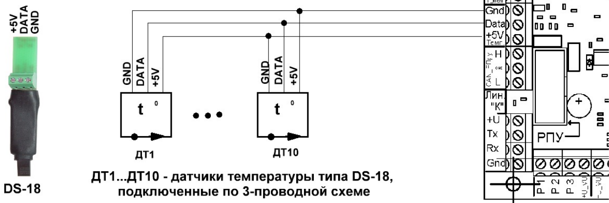
Рисунок П4 - Схема подключения ТМ, микрофона, датчиков температуры.
